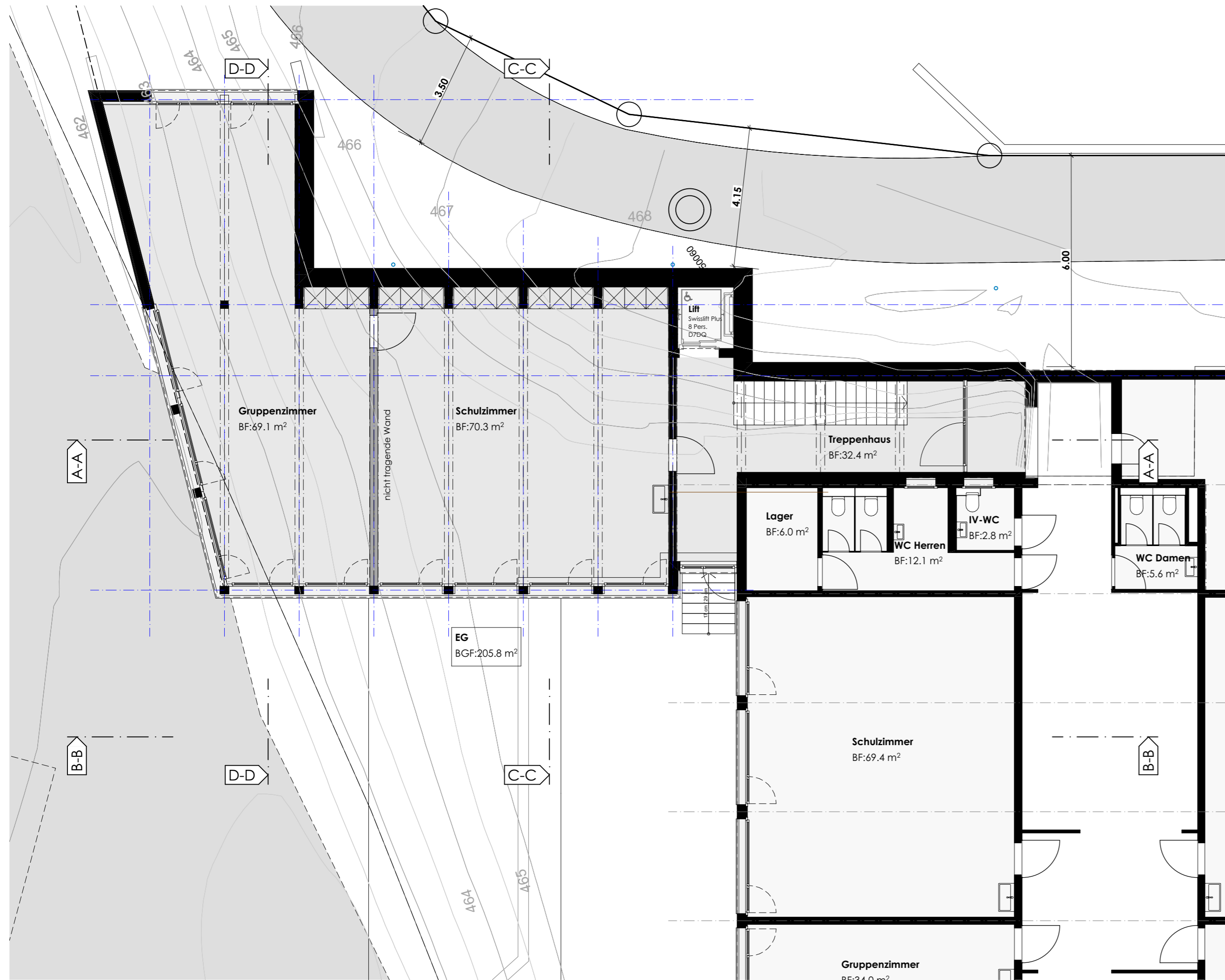
Grundriss Erdgeschoss
